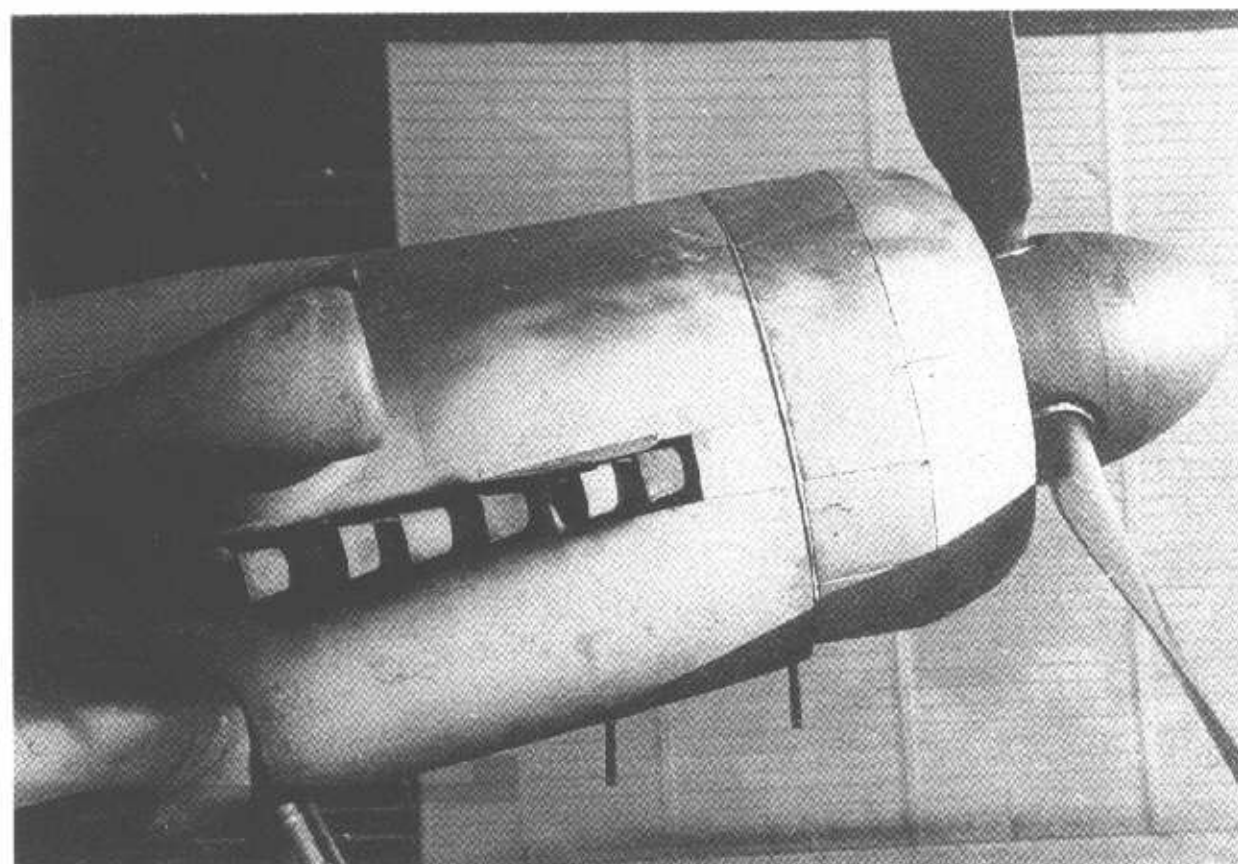
Jumo 213E mit Ladeluftkühler
